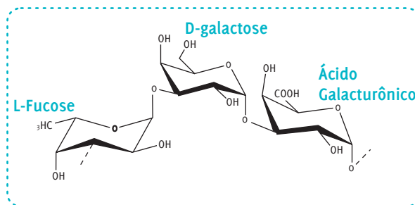
Fig. 1: Estrutura do Fucogel®
