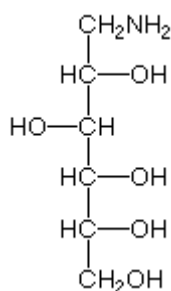
Figura 1. Estrutura química de Glucamina, Aminodeoxy glucitol ou Desamina® .
