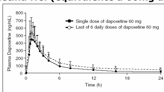
Figura 3: Perfis da concentração plasmática após dose única e múltipla de Dapoxetina HCl (equivalente a 60mg da base).
